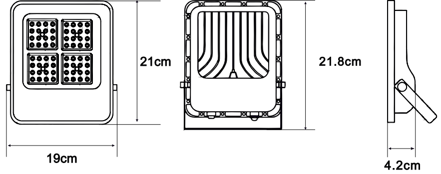
Teknik Çizim / Technical Drawing
