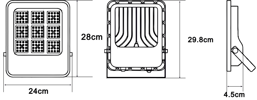
Teknik Çizim / Technical Drawing
