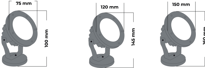
Teknik Çizim / Technical Drawing
